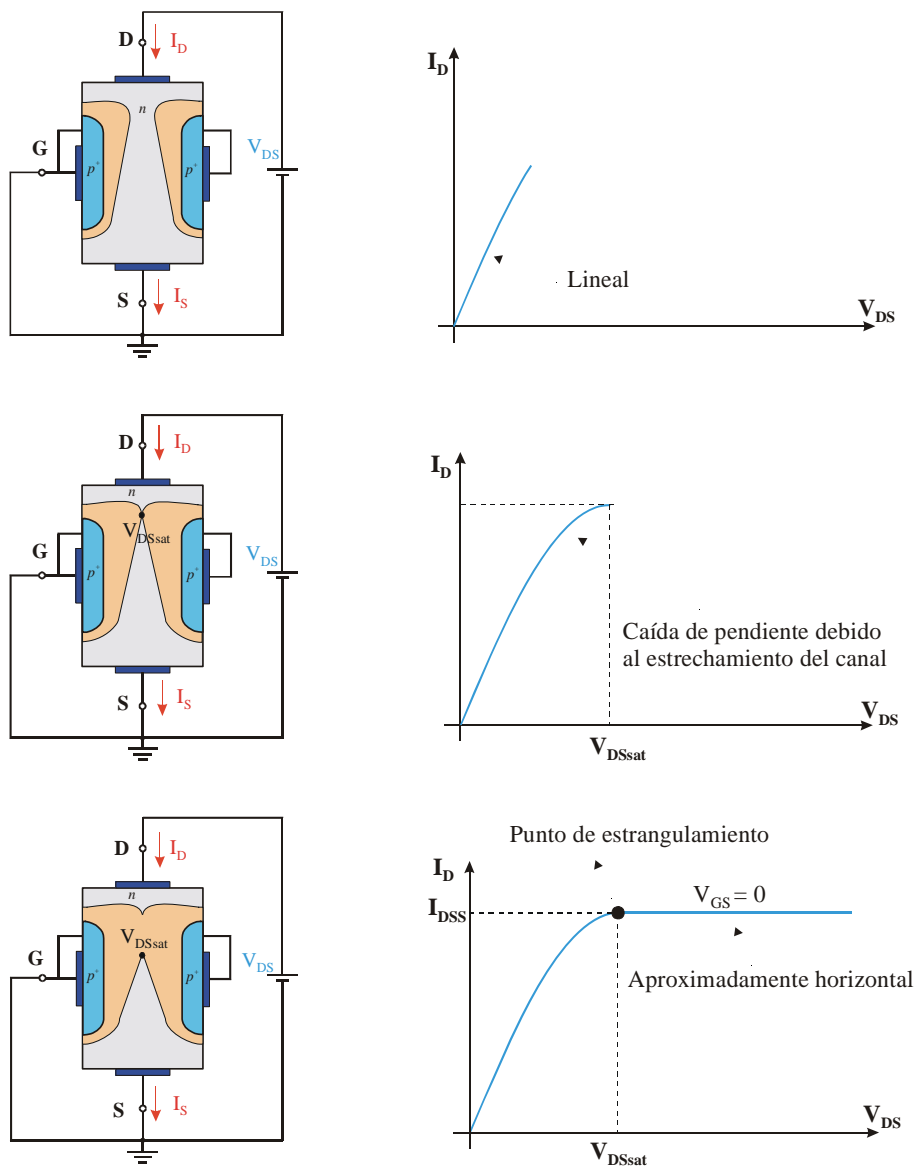
Figura 4.5.- Característica I_D - V_{DS} con V_{GS} = 0 .
