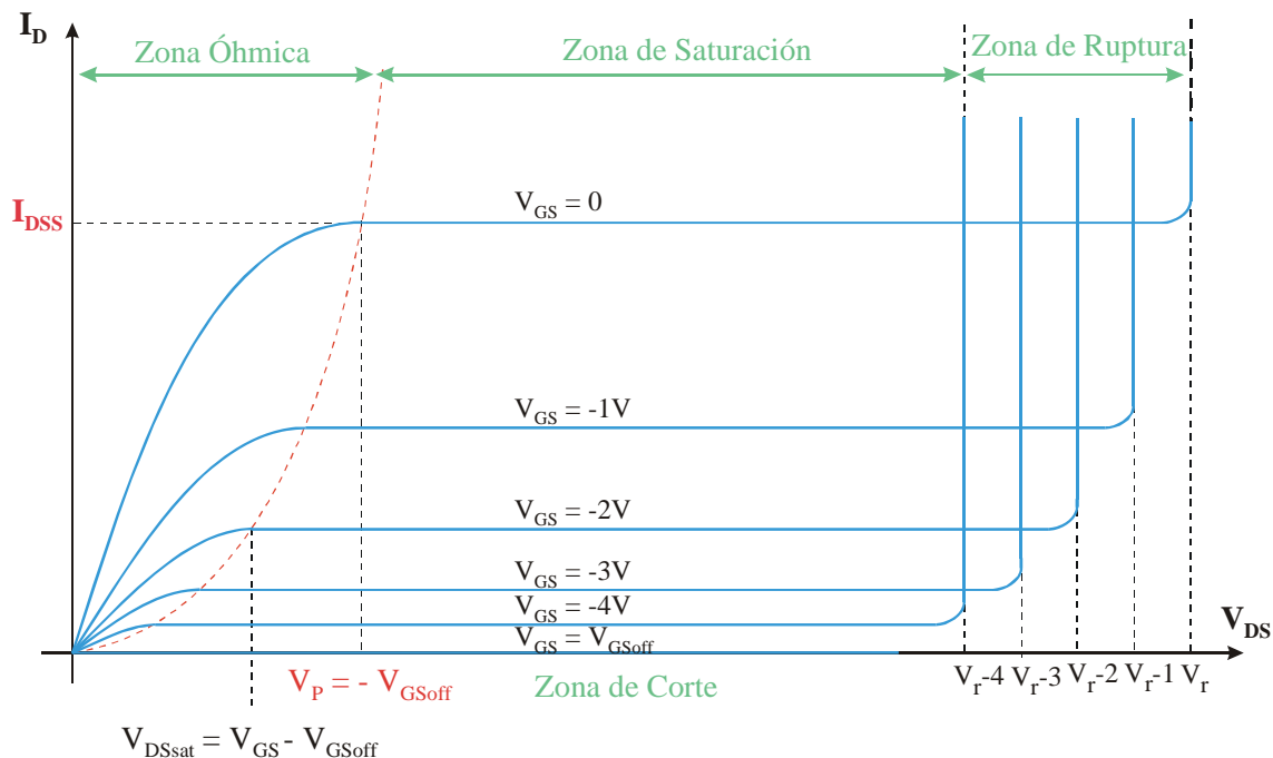
Figura 4.9.- Características ideales de un JFET de canal n.
