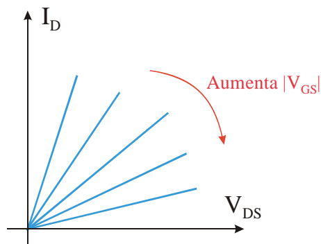
Figura 4.8.- La tensión V_{GS} modula la anchura del canal. El dispositivo se comporta como una resistencia controlada por V_{GS} .
