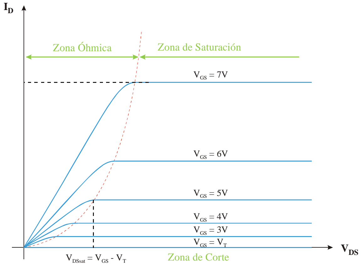
Figura 4.21.- Características ideales de un MOSFET de acumulación canal n.
