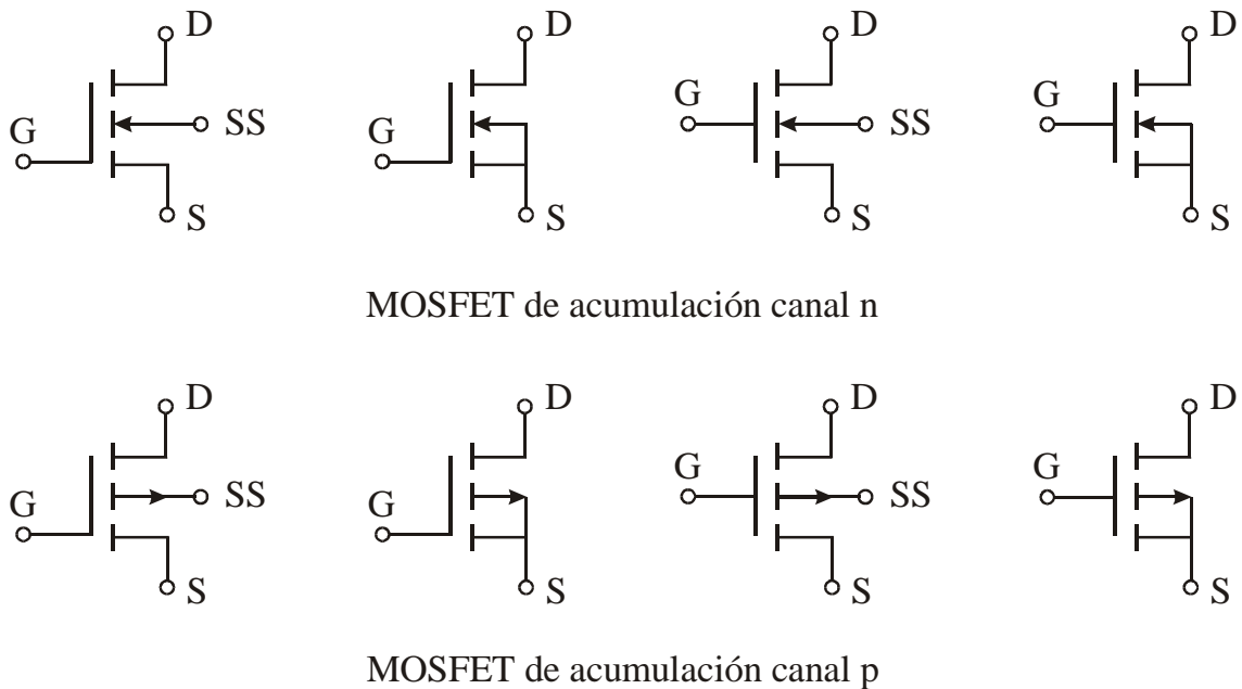
Figura 4.14.- Símbolos del MOSFET de acumulación
