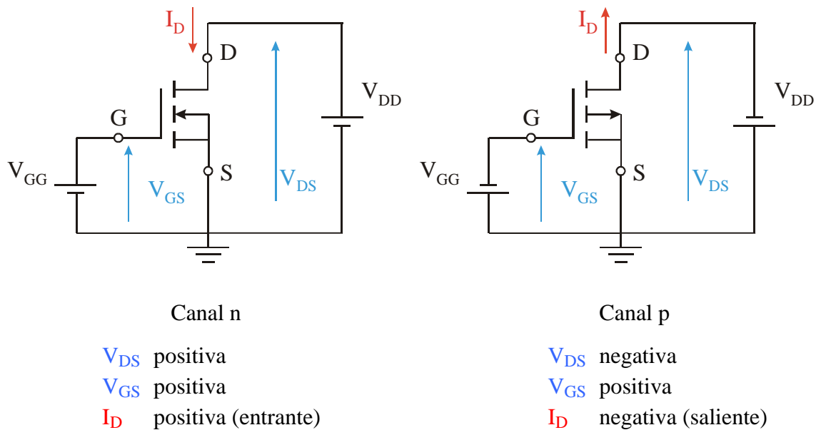
Figura 4.15.- Polarización del MOSFET de acumulación.
