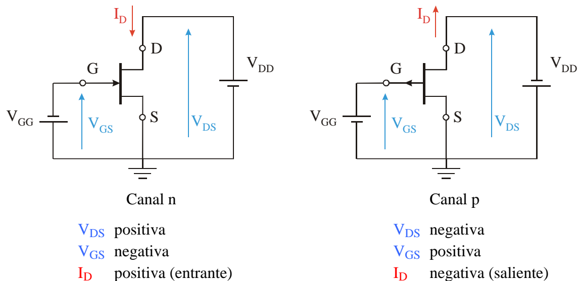
Figura 4.3.- Polarización del JFET.
