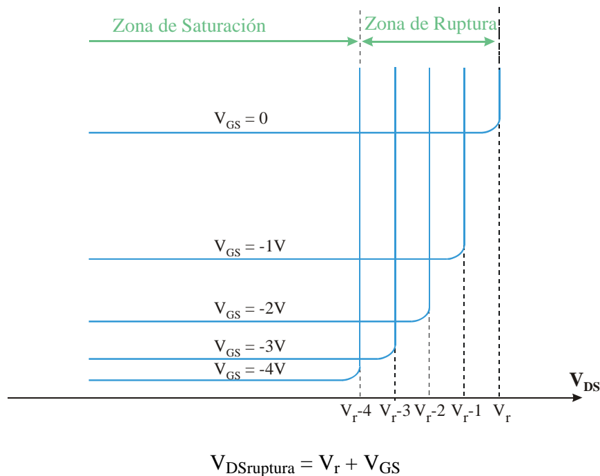
Figura 4.12.- Zona de ruptura. Las líneas correspondientes a los distintos valores de V_{GS} se cruzan.
