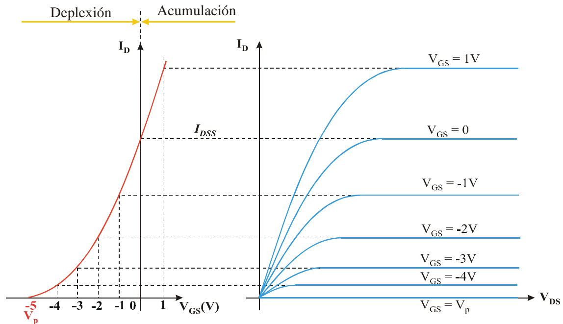
Figura 4.28.- Características ideales de un MOSFET de deplexión canal n.
