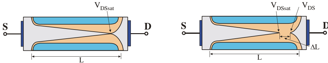
Figura 4.6.- JFET de canal largo. Para tensiones superiores a V_{DSsat} el exceso de tensión cae en la zona de canal vaciado \Delta L .
