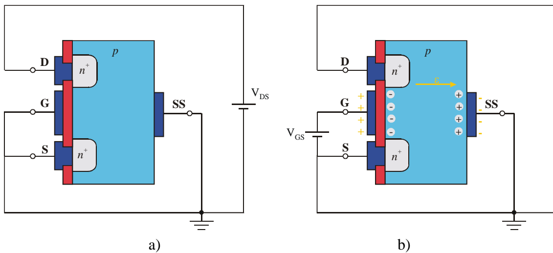
Figura 4.16.- Efecto de V_{GS} ; a) V_{GS} = 0 b) V_{GS} > 0 .
