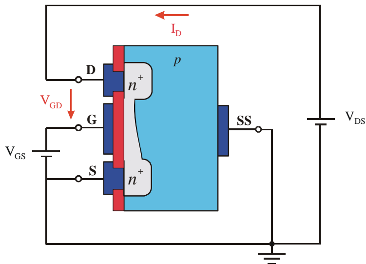
Figura 4.19.- Efecto de la tensión V_{DS} . El canal se estrecha más de la zona del drenador.
