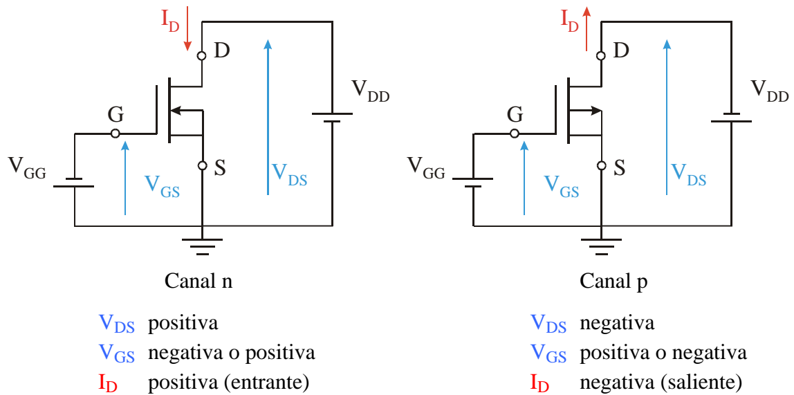
Figura 4.26.- Polarización del MOSFET de deplexió.
