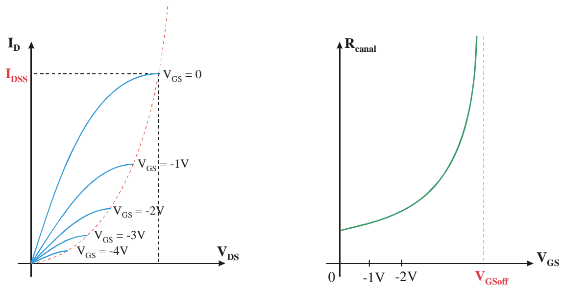
Figura 4.10.- Para V_{DS} < V_{DSsat} el JFET se comporta como una resistencia variable con V_{GS} .
