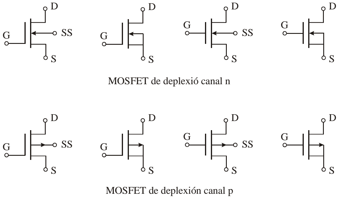
Figura 4.25.- Símbolos del MOSFET de deplexió.
