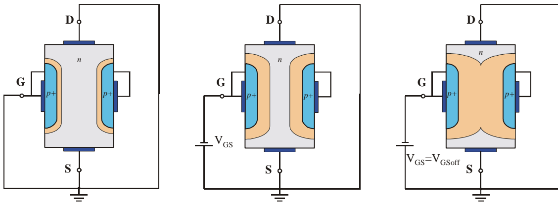
Figura 4.7.- La tensión V_{GS} modula la anchura del canal. Cuando V_{GS} = V_{GSoff} el canal se cierra por completo
