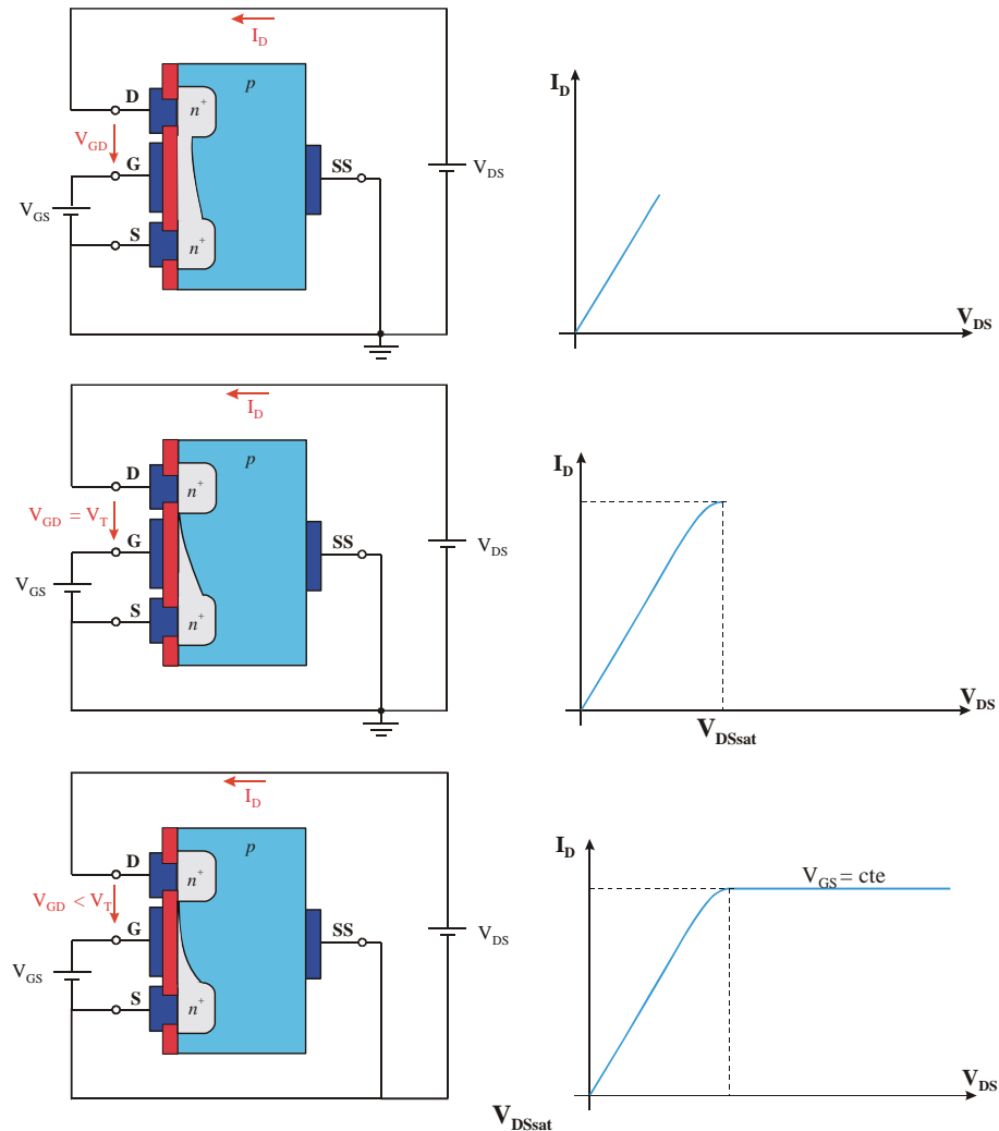
Figura 4.20.- Característica I_D - V_{DS} para una valor de V_{GS} constante.
