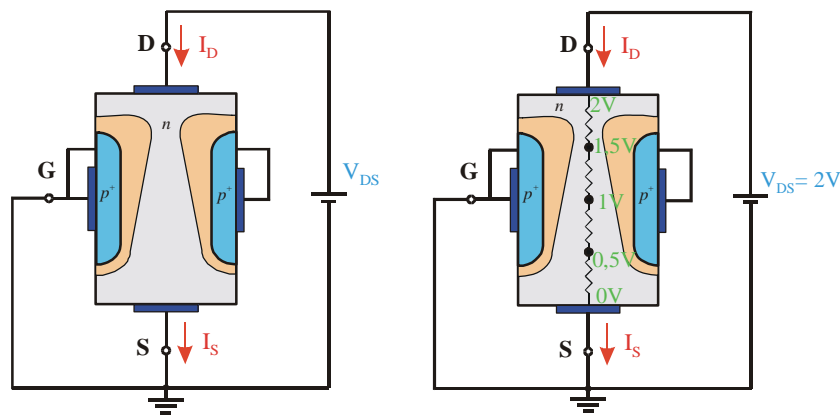
Figura 4.4.- Efecto de la tensión V_{DS} . El canal se estrecha de la zona del drenador.
