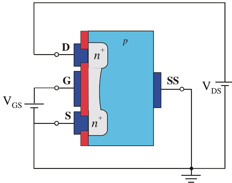
Figura 4.27.- Funcionamiento del MOSFET de depleción canal n.
