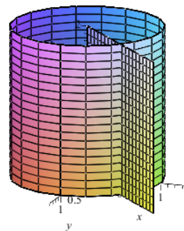
\theta constante y r constante
