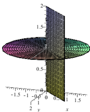
\theta constante y z constante
